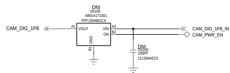
CAMERA VDDIO - 1.8V
